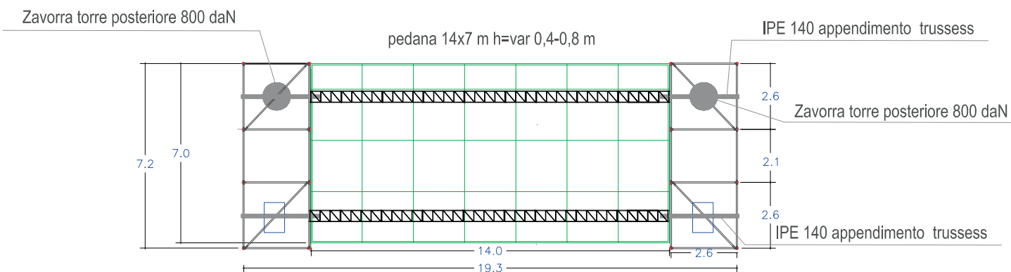
PIANTA
